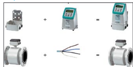
4 pav. Elektromagnetinio debitomačio distancinė versija
